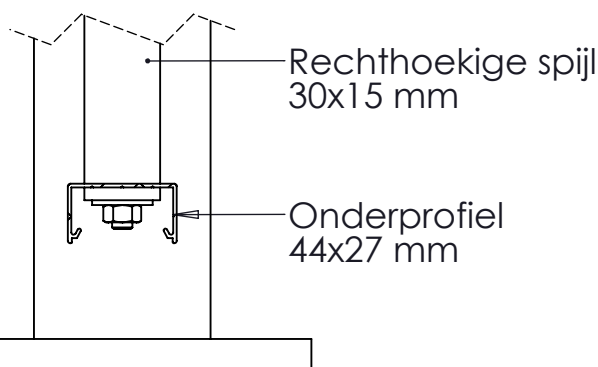
SECTION A-A SCALE 1 : 3
